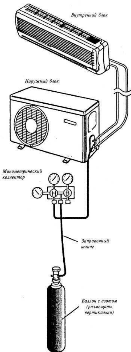
Рис. 13. Опрессовка контура циркуляции хладагента
