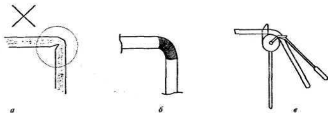
Рис. 12. Выполнение сгиба трубки: а - неправильное; б - с помощью пружины; в - с помощью трубогиба
