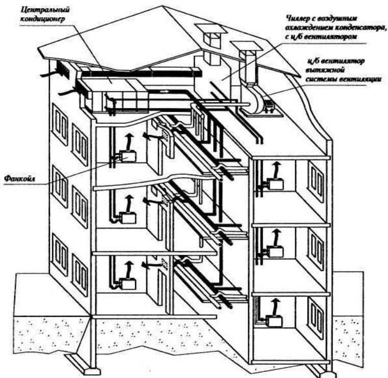
Рис. 4. Система кондиционирования воздуха офисного здания на базе центрального кондиционера и чиллер-фанкойлов
