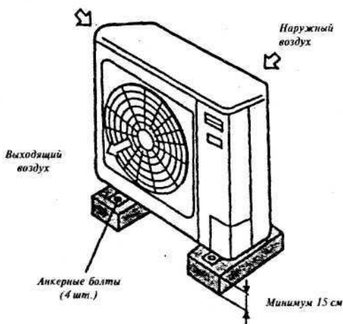
Рис. 8. Размещение наружного блока на опорах
