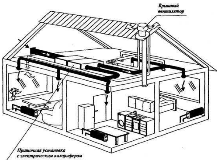
Рис. 1. Система приточно-вытяжной вентиляции жилого одноэтажного дома
