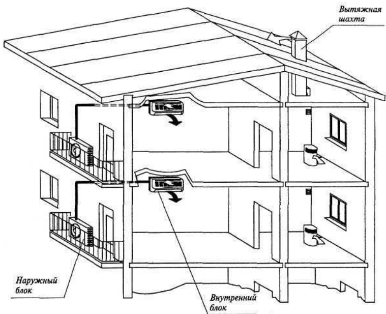
Рис. 2. Применение сплит-систем в помещениях жилого дома
