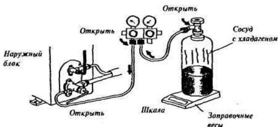
Рис. 16. Заправка с использованием заправочных весов
