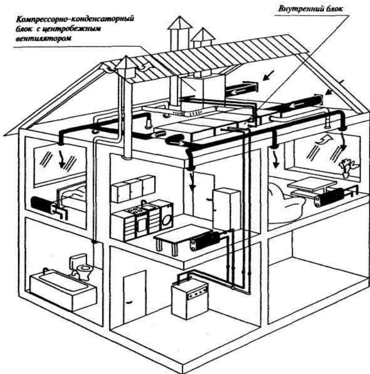
Рис. 3. Система кондиционирования воздуха коттеджа
