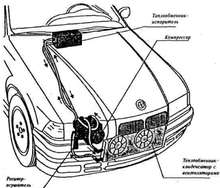
Рис. 5. Основные элементы автомобильной климатической системы
