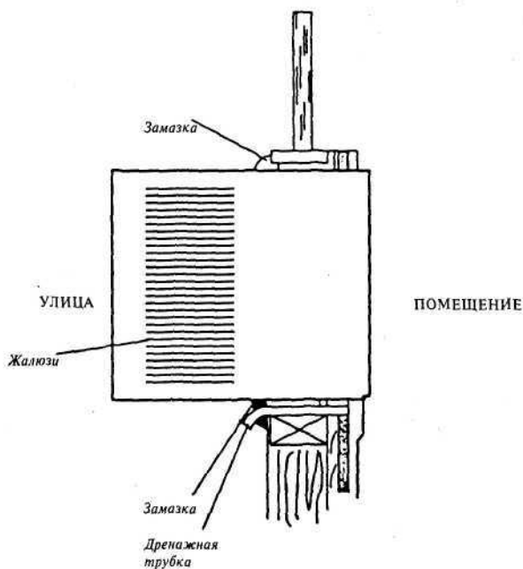
Рис. 6. Уплотнение при установке оконного кондионера
